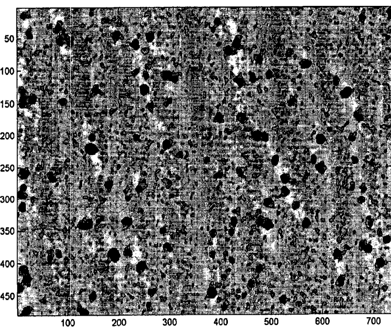
图 4: 在 R_k 构造中的点 D 高度处取阈值的图像 (10x 放大下的干涉仪图像)。
