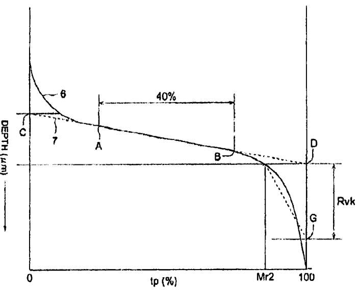
图 3: R_k 构造。
