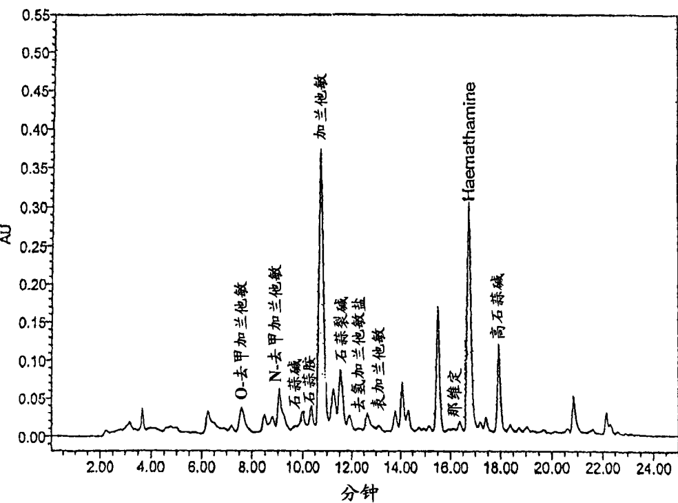
图 2. 实施例 1 获得的初级提取物的 HPLC 分析
