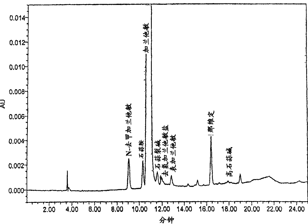
图 5. 实施例 1 获得的盐酸加兰他敏的 HPLC 分析
