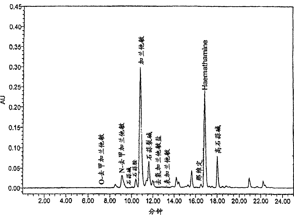
图 3. 实施例 1 获得的粗生物碱浓缩物的 HPLC 分析
