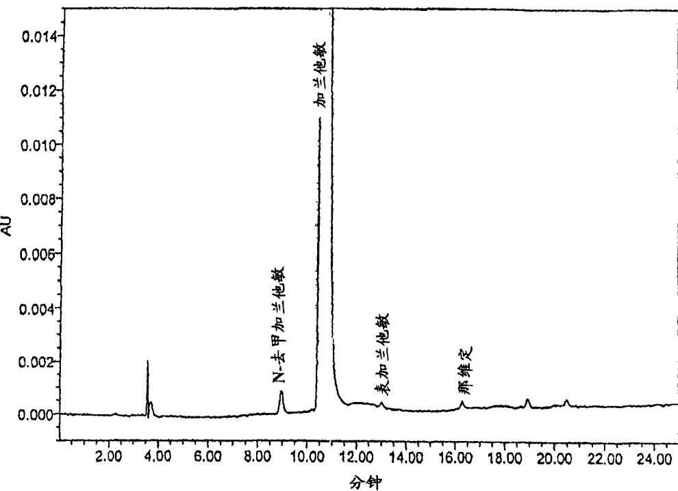
图 7. 实施例 2 获得的加兰他敏的碱的 HPLC 分析
