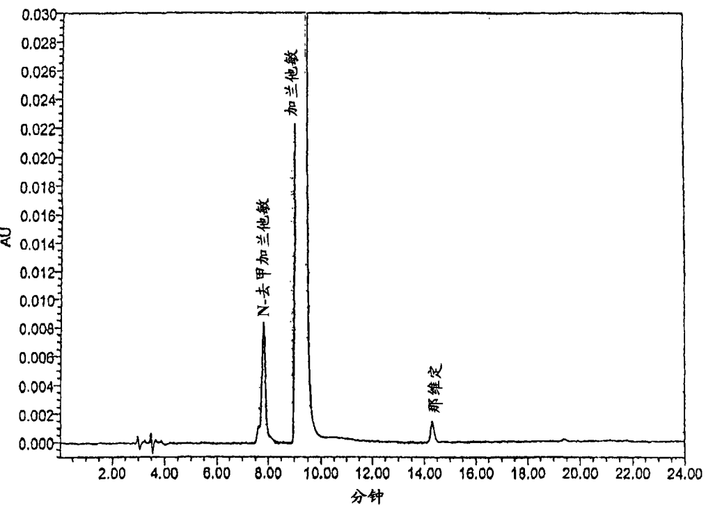
图 9. 实施例 3 获得的加兰他敏的碱的 HPLC 分析
