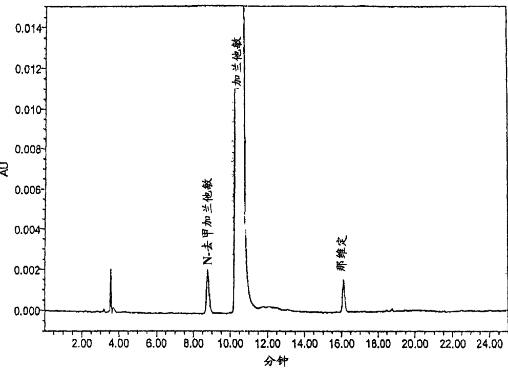
图 6. 实施例 1 获得的加兰他敏的碱的 HPLC 分析
