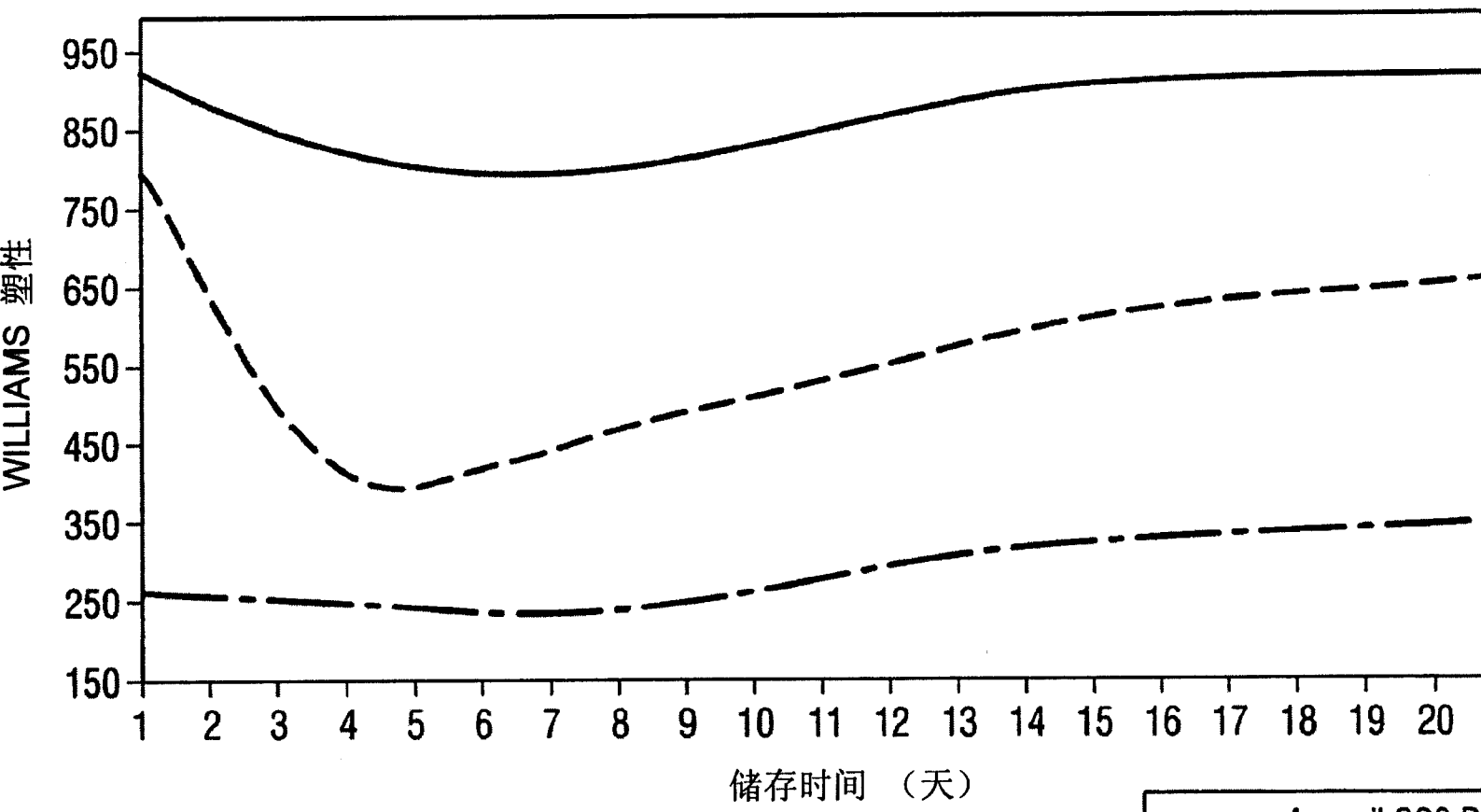
图 2 VP 3744 皱皮硬化曲线
