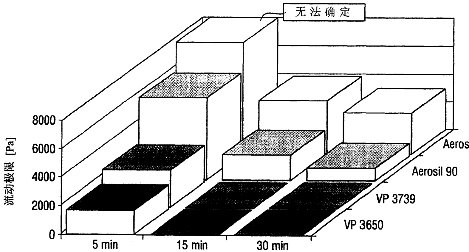
图 5 20%二氧化硅在分散 5、15、30 分钟后的流动极限
