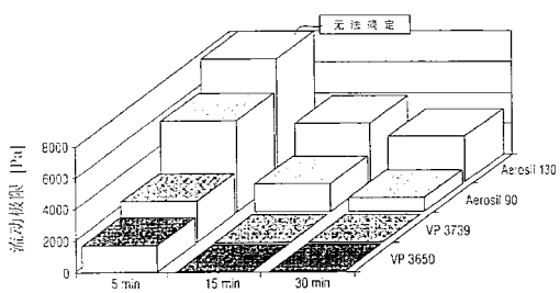
20%二氧化硅在分散 5、15、30 分钟后的流动极限
