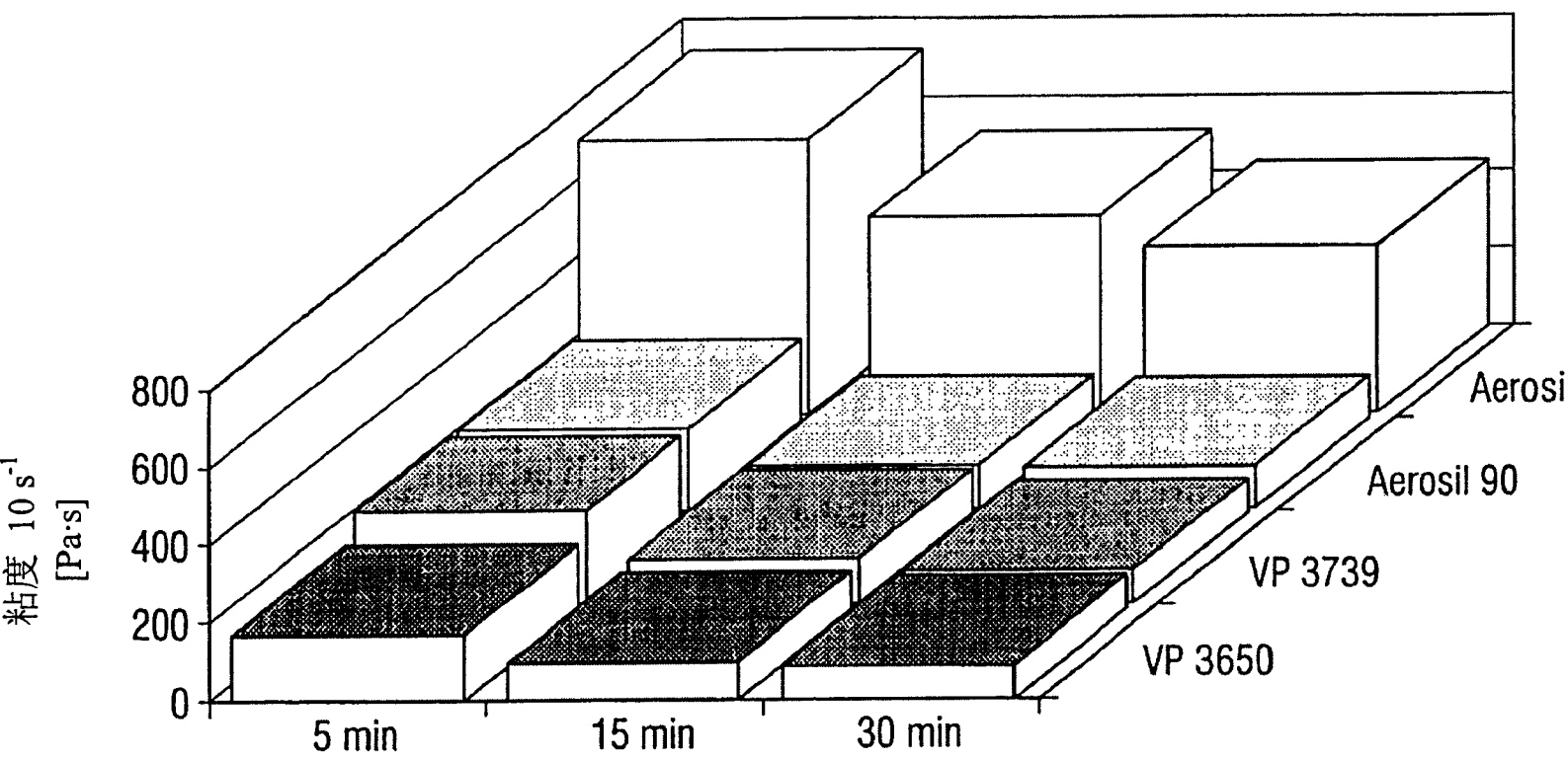
图 3 15%二氧化硅在分散 5、15、30 分钟后的粘度
