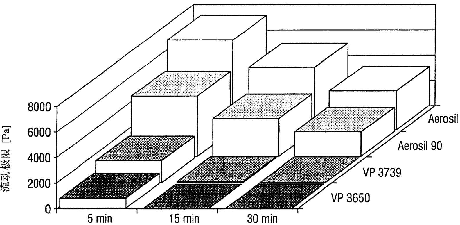
图 4 15%二氧化硅在分散 5、15、30 分钟后的流动极限
